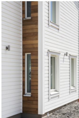
J KNOTBRÄDA STANDARD Grund och mellanstruken, vit. 28x145 mm / 28x170 mm Tillval utan kostnad: 21x70 - 145 mm/21x95 - 170 mm
